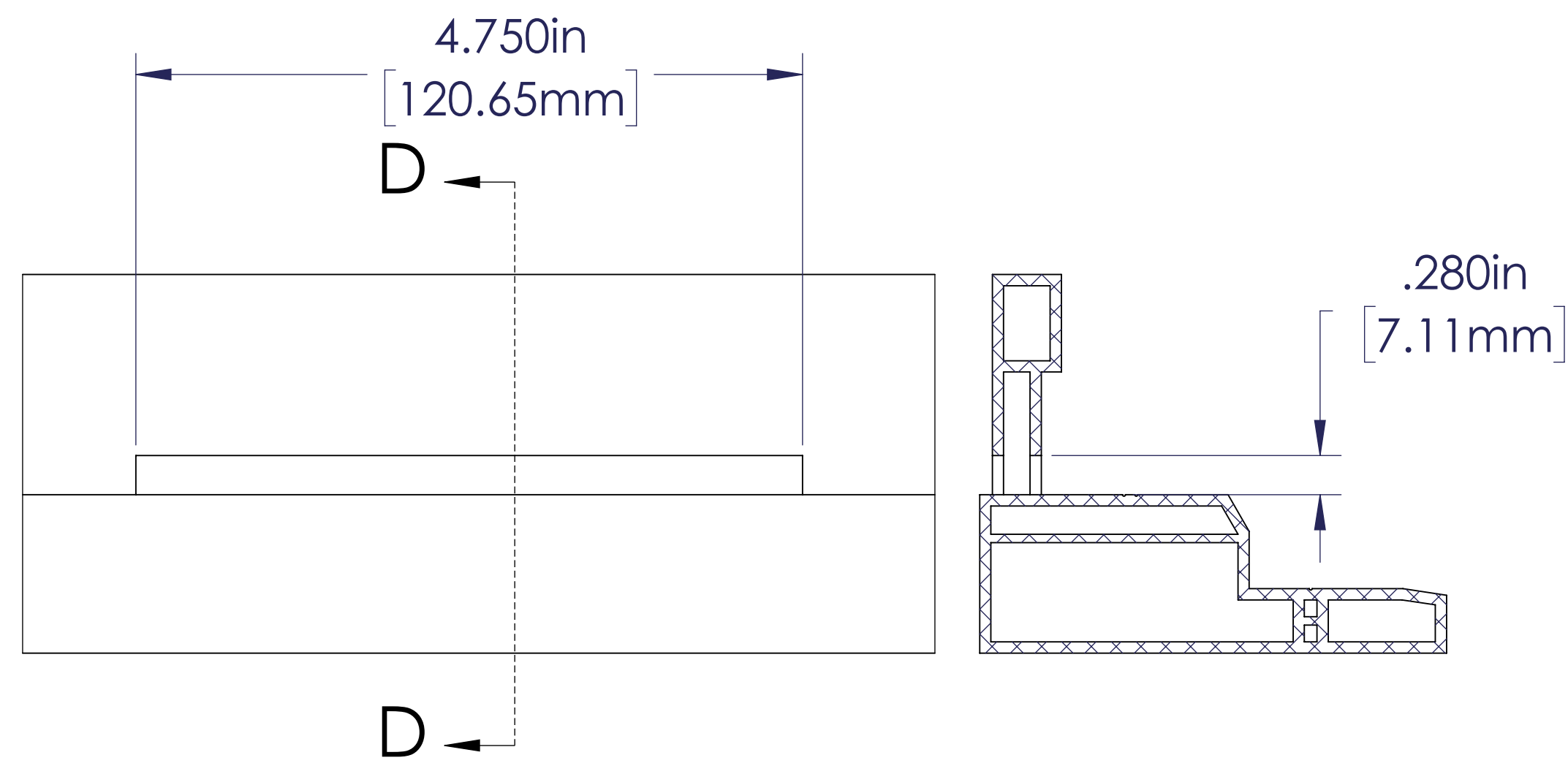
SECTION D-D SCALE 1 : 1
