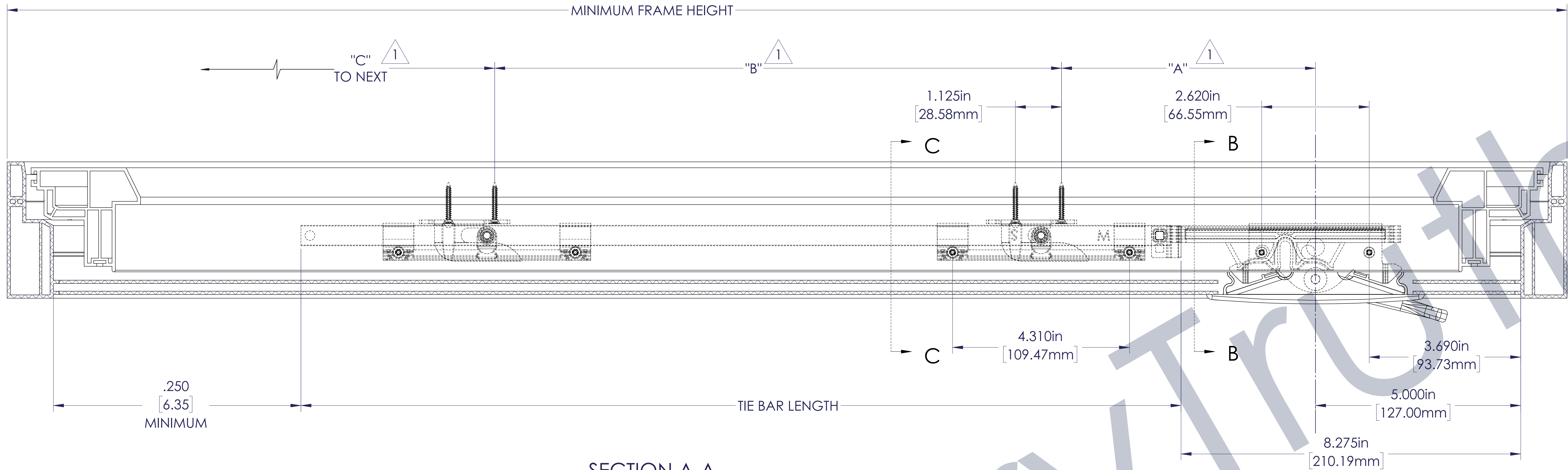
SECTION A-A SCALE 1 : 1
